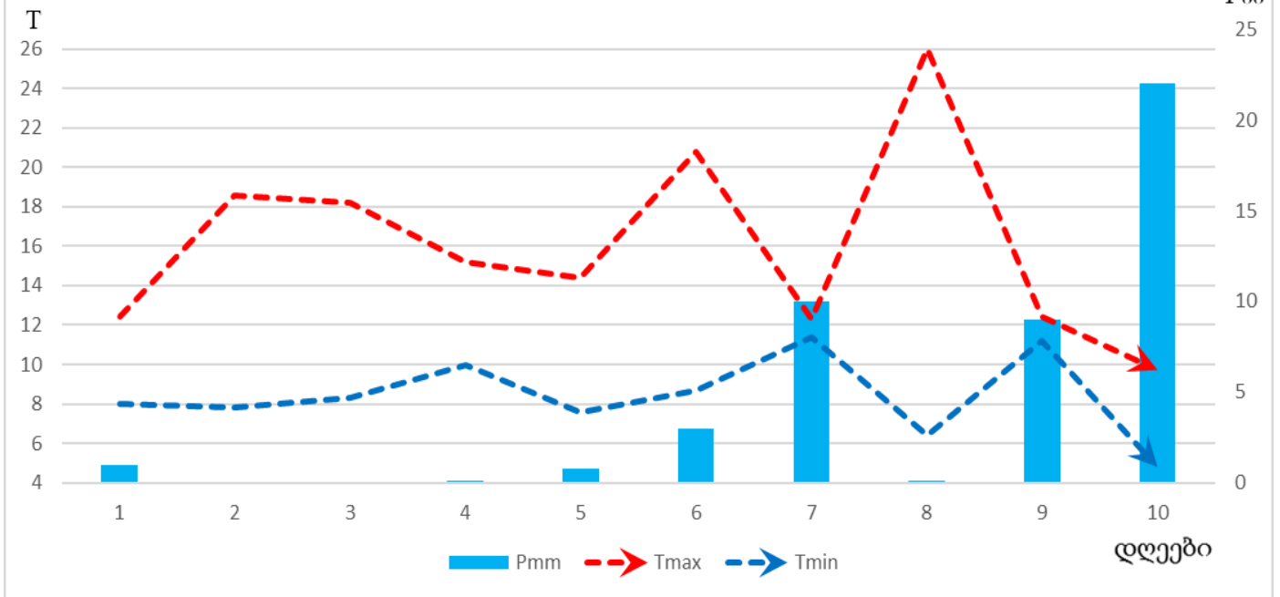
ჰაერის ტემპერატურის (T) და ნალექების (Pმმ) მსვლელობა ზუგდიდში მარტის III დეკადაში
