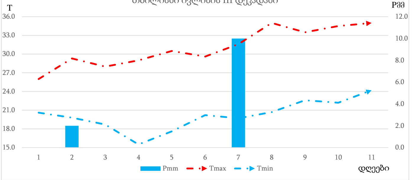
ჰაერის ტემპერატურის (T) და ნალექების (Pmm) მსვლელობა თბილისში ივლისის III დეკადაში
