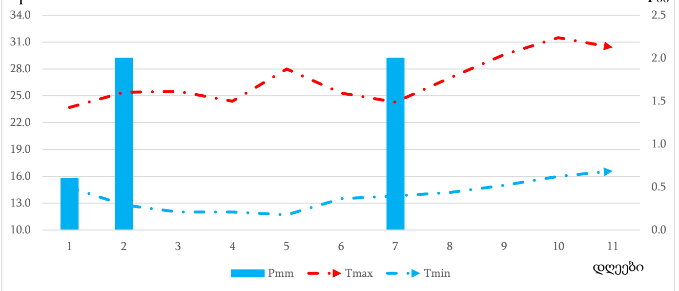
ჰაერის ტემპერატურის (T) და ნალექების (Pmm) მსვლელობა თიანეთში ივლისის III დეკადაში
