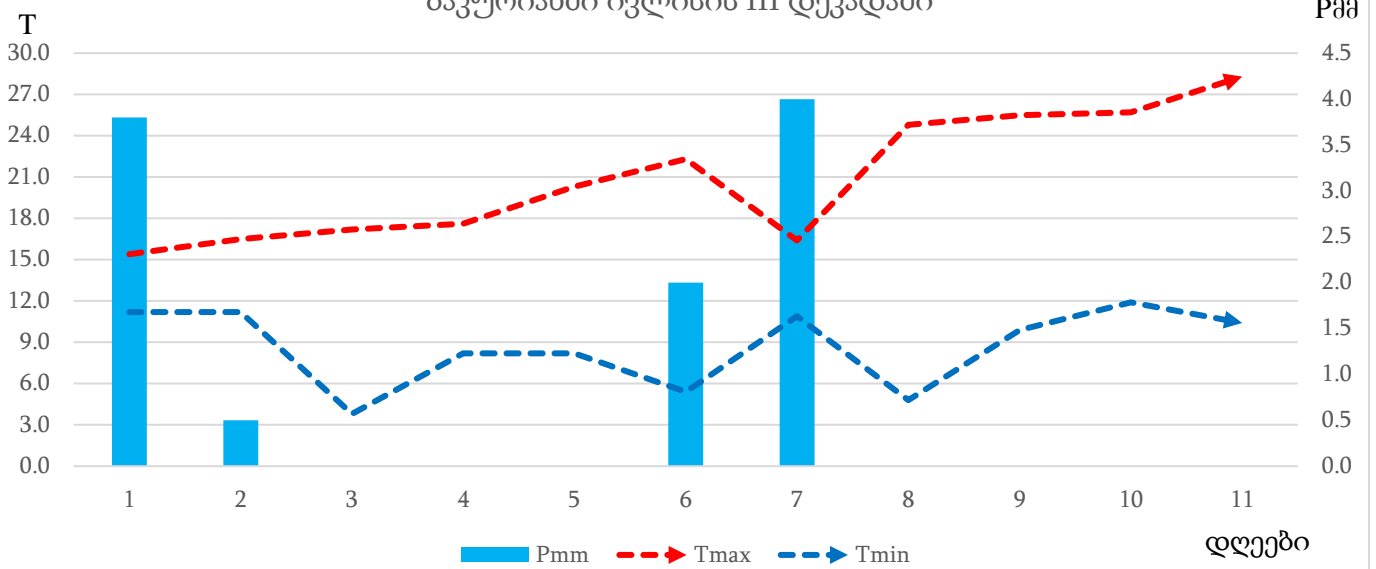
ჰაერის ტემპერატურის (T) და ნალექების (Pmm) მსვლელობა ბაკურიანში ივლისის III დეკადაში
