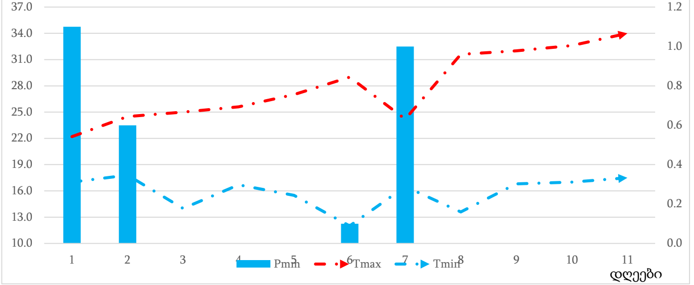
ჰაერის ტემპერატურის (T) და ნალექების (Pmm) მსვლელობა გორში ივლისის III დეკადაში
