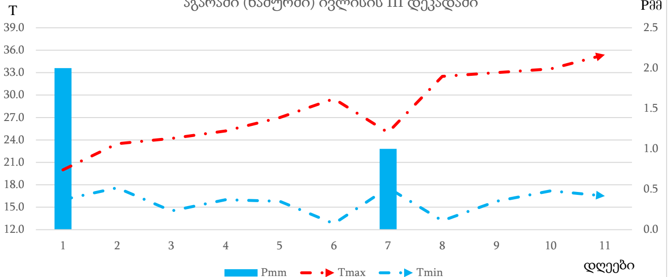
ჰაერის ტემპერატურის (T) და ნალექების (Pmm) მსვლელობა აგარაში (ხაშურში) ივლისის III დეკადაში
