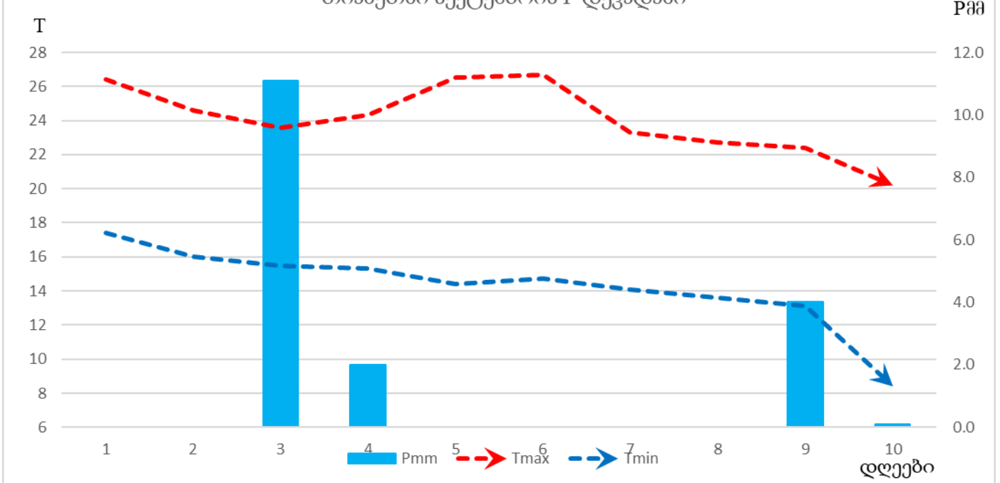
ჰაერის ტემპერატურის (T) და ნალექების (Pმმ) მსვლელობა თიანეთში სექტემბრის I დეკადაში
