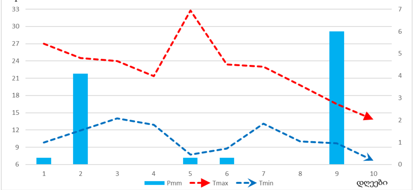
ჰაერის ტემპერატურის (T) და ნალექების (Pმმ) მსვლელობა ბაკურიანში სექტემბრის I დეკადაში
