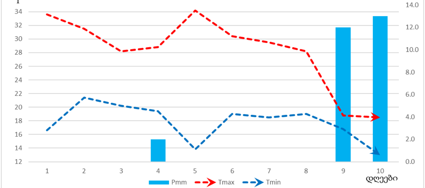
ჰაერის ტემპერატურის (T) და ნალექების (Pმმ) მსვლელობა აგარაში (ხაშური) სექტემბრის I დეკადაში
