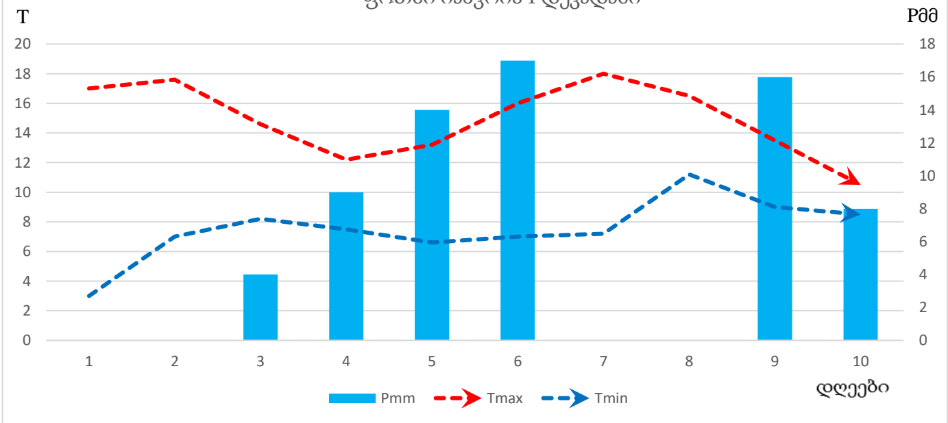
ჰაერის ტემპერატურის (T) და ნალექების (Pმმ) მსვლელობა ფოთში იანვრის I დეკადაში
