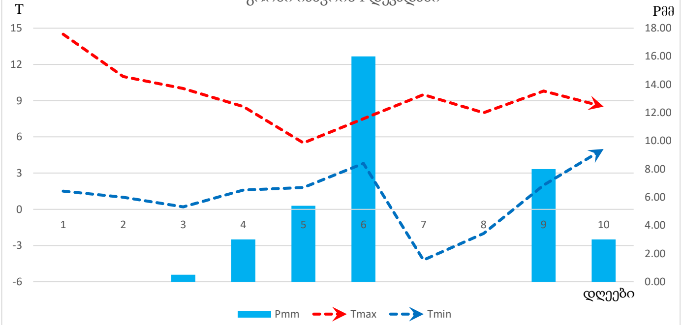
ჰაერის ტემპერატურის (T) და ნალექების (Pმმ) მსვლელობა გორში იანვრის I დეკადაში
