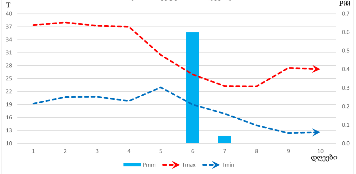
ჰაერის ტემპერატურის (T) და ნალექების (Pმმ) მსვლელობა თბილისში სექტემბრის I დეკადაში
