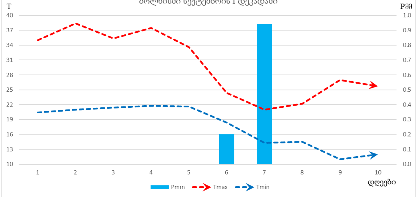
ჰაერის ტემპერატურის (T) და ნალექების (Pმმ) მსვლელობა ზოლნისში სექტემბრის I დეკადაში
