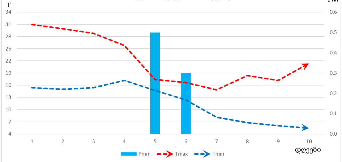
ჰაერის ტემპერატურის (T) და ნალექების (Pმმ) მსვლელობა მთა საბუეთში სექტემბრის I დეკადაში
