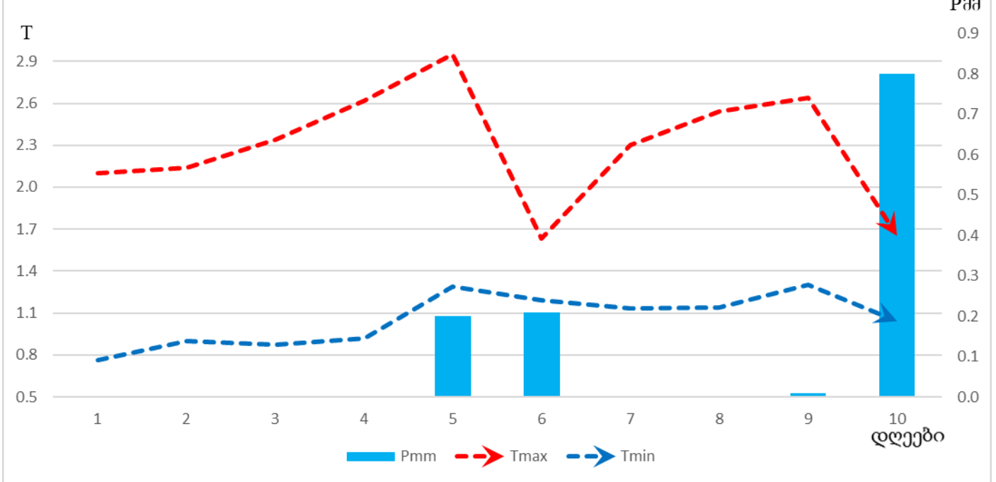
ჰაერის ტემპერატურის (T) და ნალექების (Pმმ) მსვლელობა თბილისში მაისის II დეკადაში
