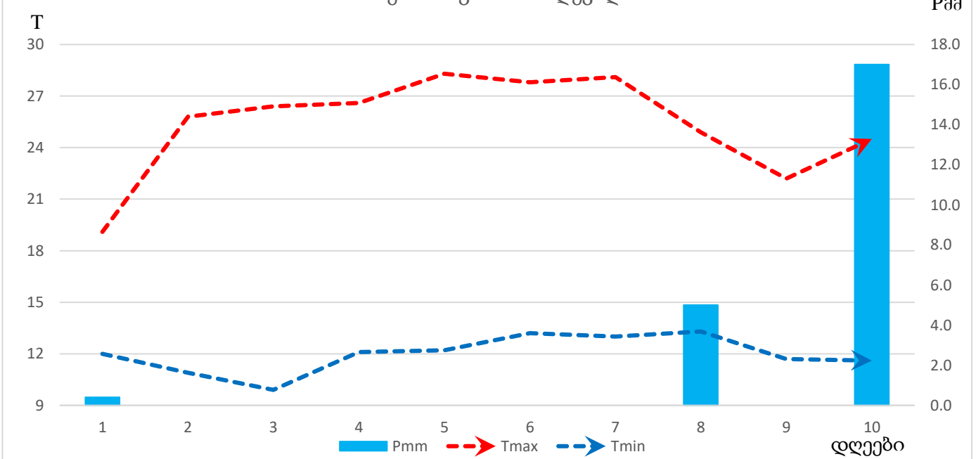
ჰაერის ტემპერატურის (T) და ნალექების (Pმმ) მსვლელობა თიანეთში ივნისის I დეკადაში
