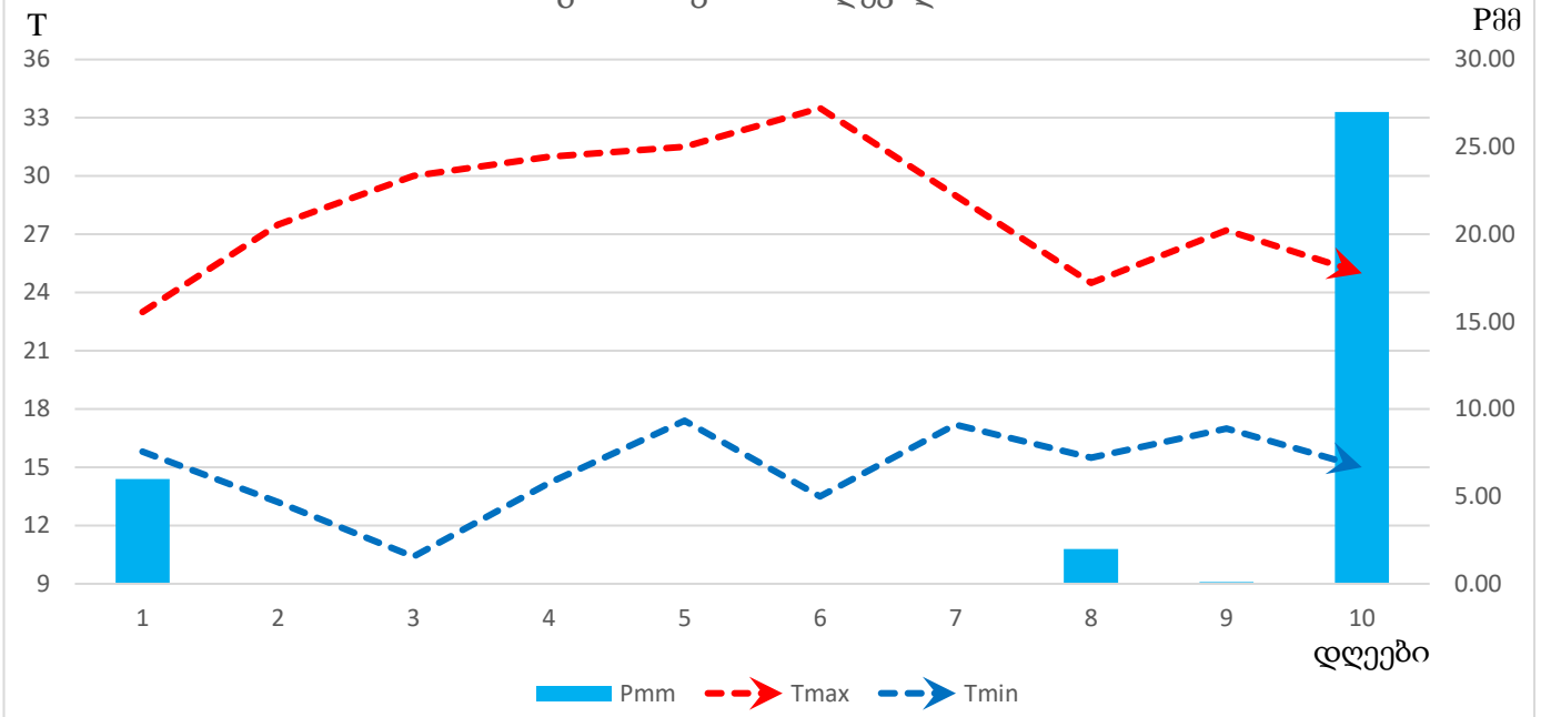
ჰაერის ტემპერატურის (T) და ნალექების (Pმმ) მსვლელობა გორში ივნისის I დეკადაში
