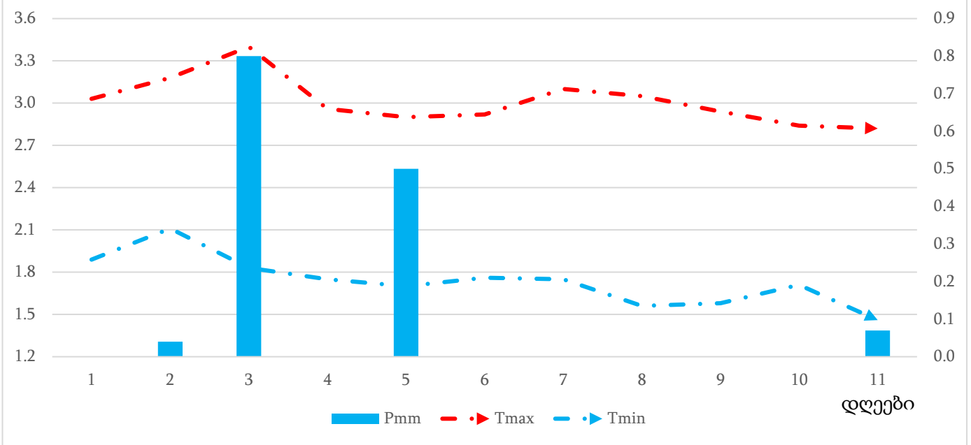
ჰაერის ტემპერატურის (T) და ნალექების (Pმმ) მსვლელობა დედოფლისწყაროში აგვისტოს III დეკადაში
