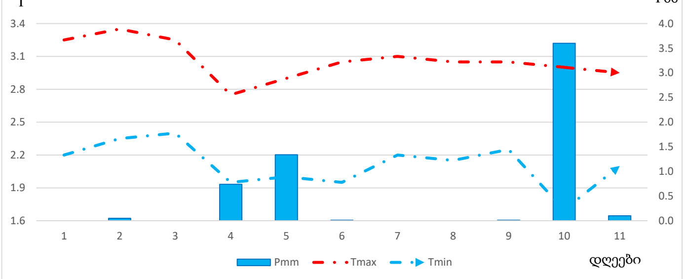
ჰაერის ტემპერატურის (T) და ნალექების (Pმმ) მსვლელობა ქობულეთში აგვისტოს III დეკადაში
