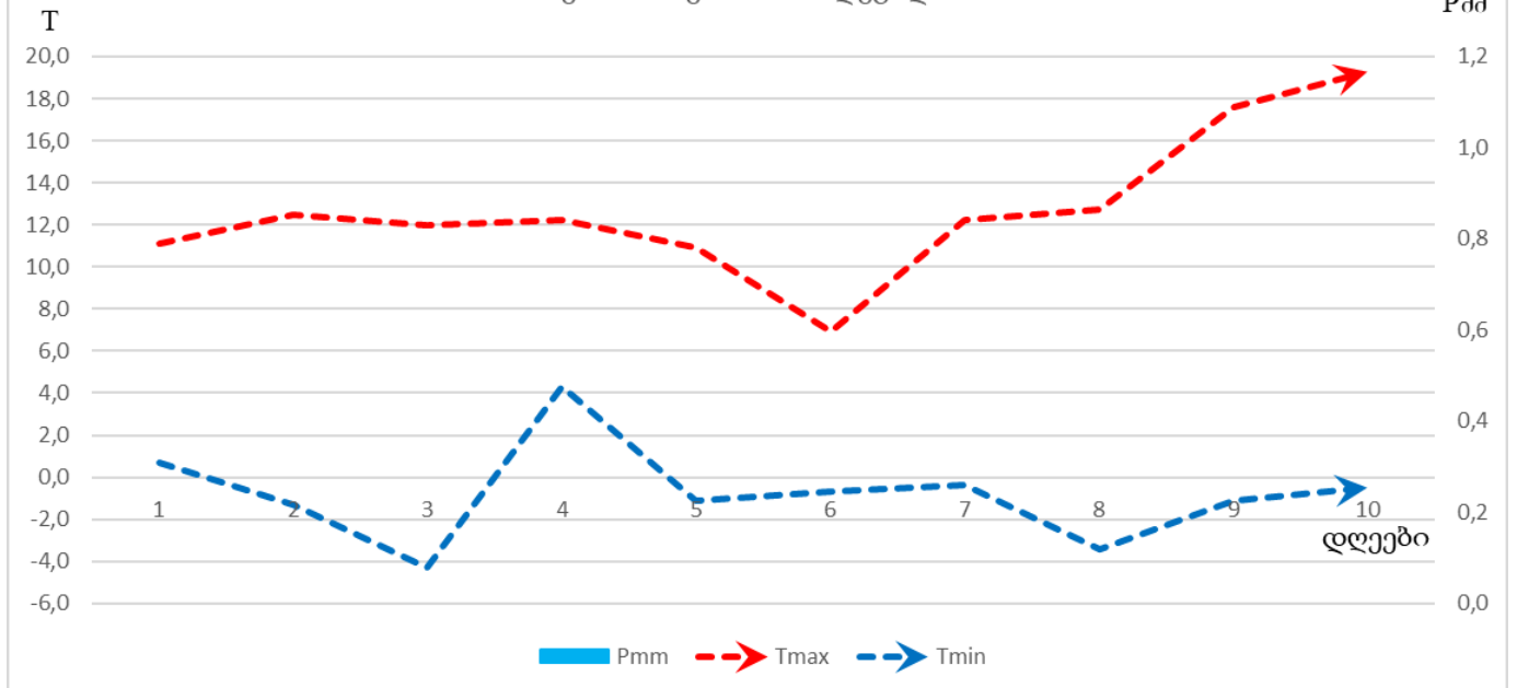
ჰაერის ტემპერატურის (T) და ნალექების (Pმმ) მსვლელობა თიანეთში ნოემბრის II დეკადაში
