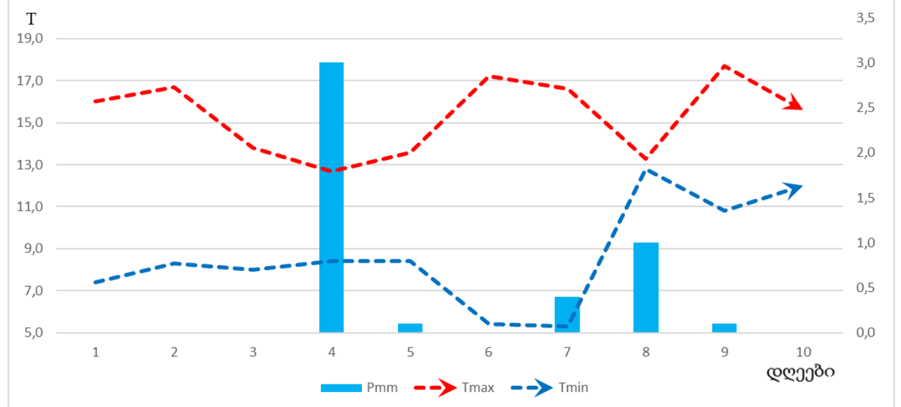
ჰაერის ტემპერატურის (T) და ნალექების (Pმმ) მსვლელობა ზუგდიდში ნოემბრის II დეკადაში
