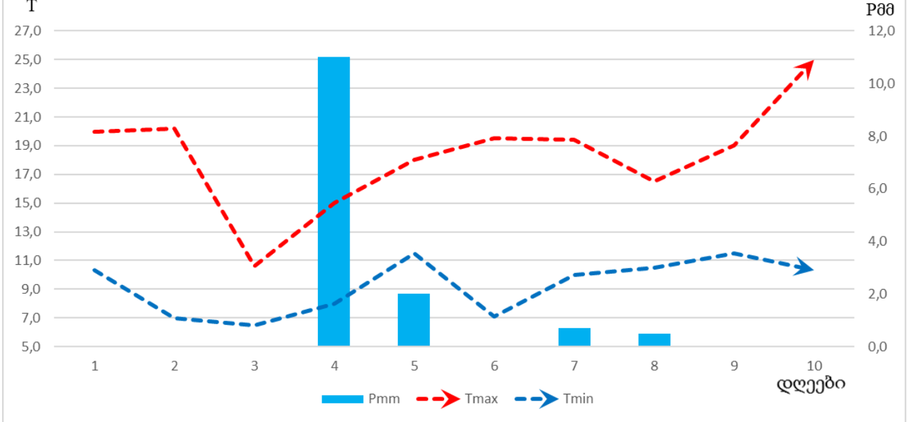
ჰაერის ტემპერატურის (T) და ნალექების (Pმმ) მსვლელობა ფოთში ნოემბრის II დეკადაში
