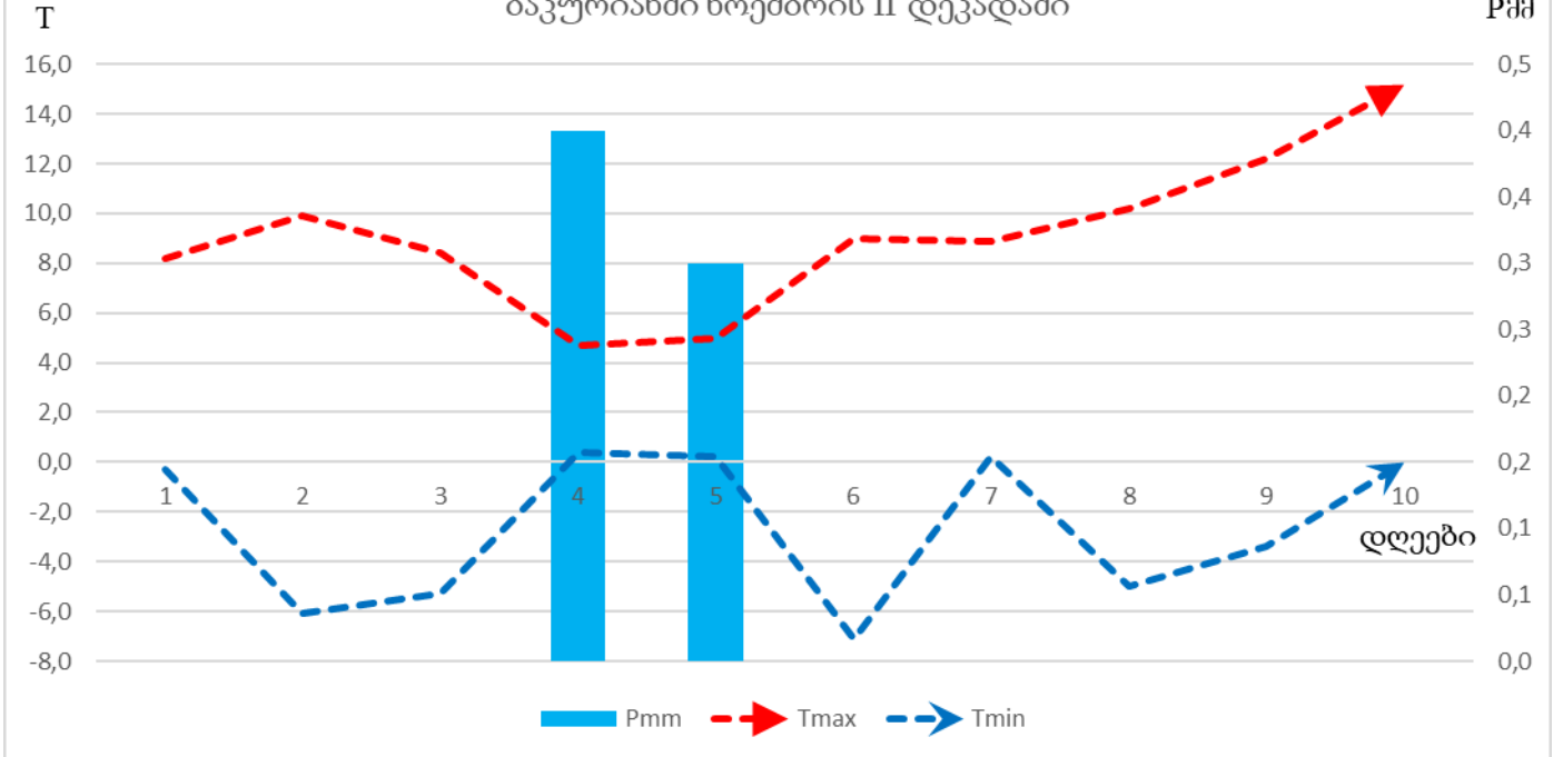
ჰაერის ტემპერატურის (T) და ნალექების (Pმმ) მსვლელობა ბაკურიანში ნოემბრის II დეკადაში
