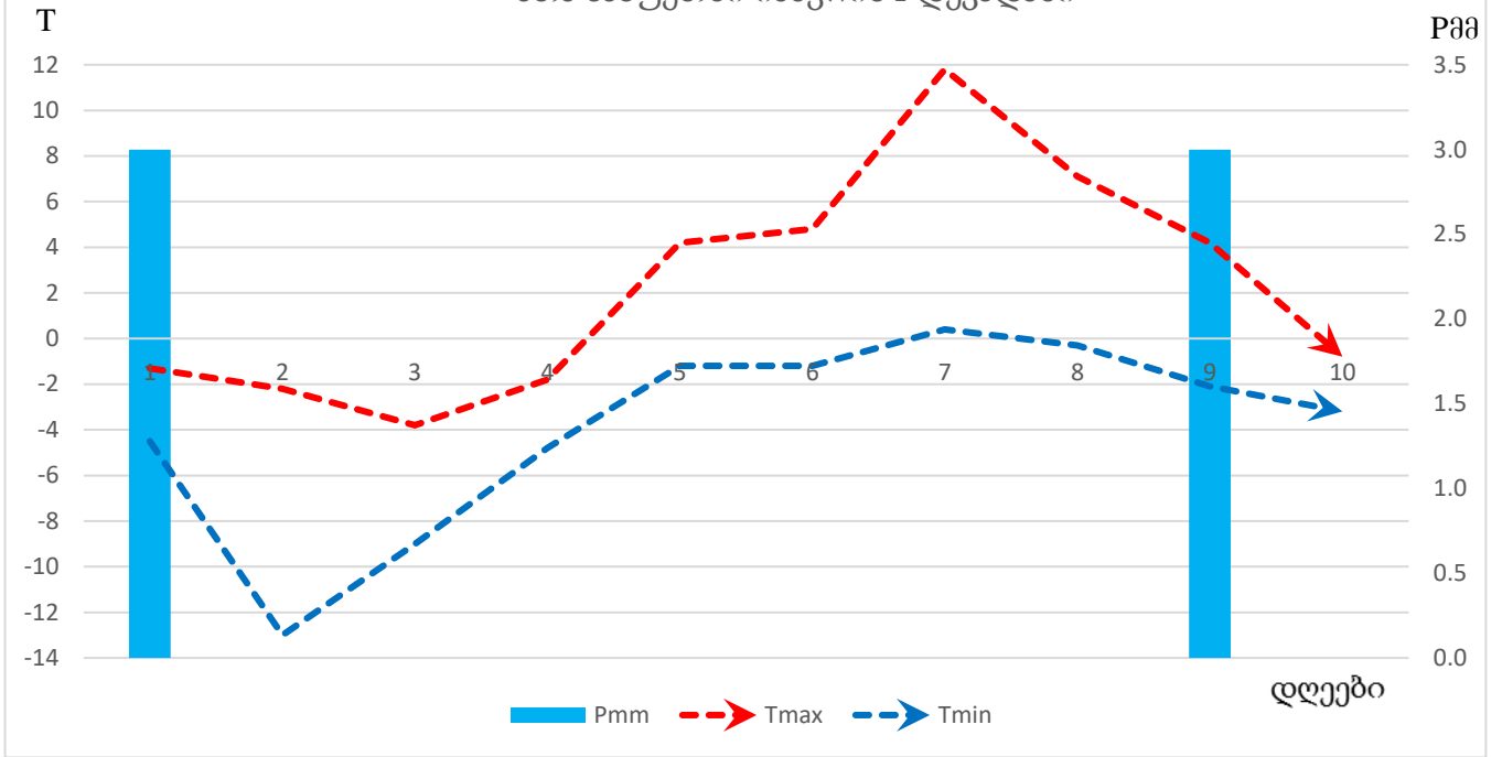
ჰაერის ტემპერატურის (T) და ნალექების (Pმმ) მსვლელობა მთა საბუეთში იანვრის I დეკადაში
