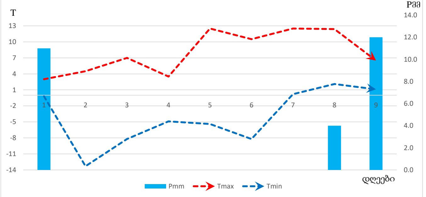
ჰაერის ტემპერატურის (T) და ნალექების (Pმმ) მსვლელობა საჩხერეში იანვრის I დეკადაში
