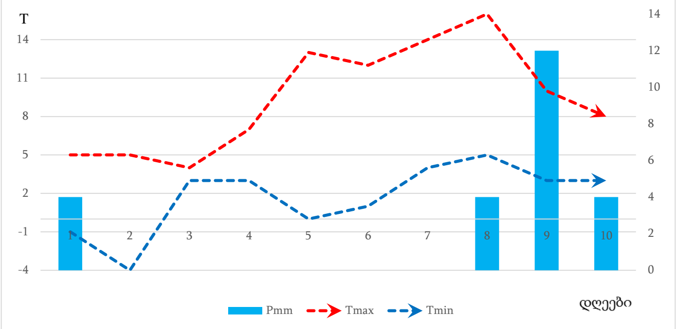
ჰაერის ტემპერატურის (T) და ნალექების (Pმმ) მსვლელობა ზესტაფონში იანვრის I დეკადაში
