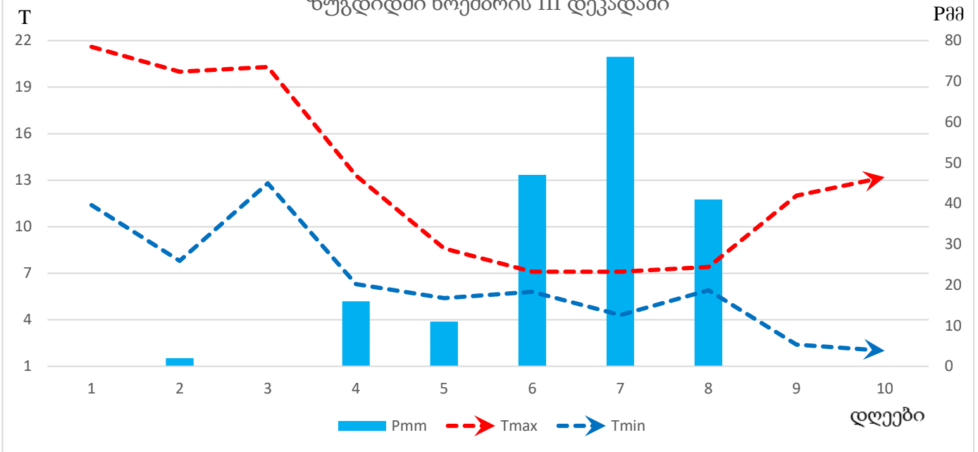
ჰაერის ტემპერატურის (T) და ნალექების (Pმმ) მსვლელობა ზუგდიდში ნოემბრის III დეკადაში
