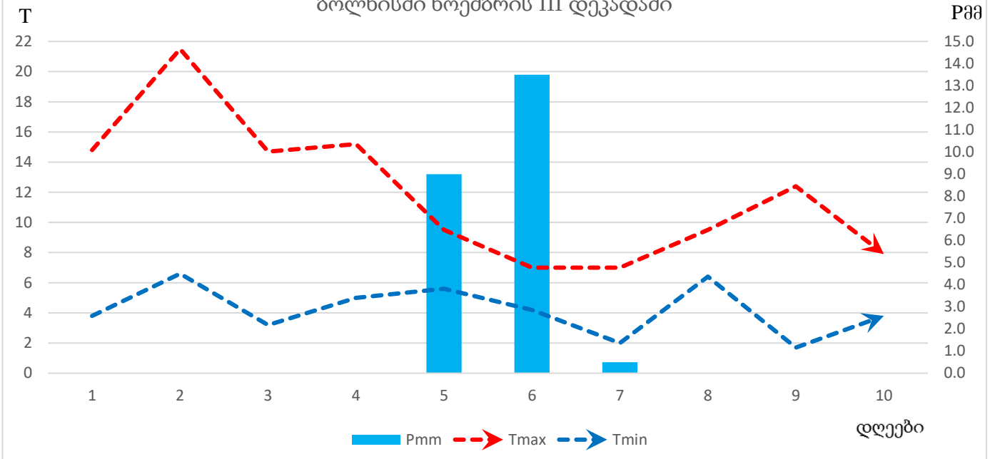
ჰაერის ტემპერატურის (T) და ნალექების (Pმმ) მსვლელობა ბოლნისში ნოემბრის III დეკადაში
