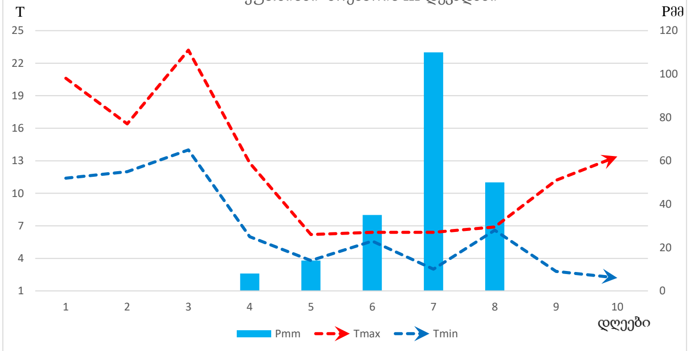
ჰაერის ტემპერატურის (T) და ნალექების (Pმმ) მსვლელობა ქუთაისში ნოემბრის III დეკადაში
