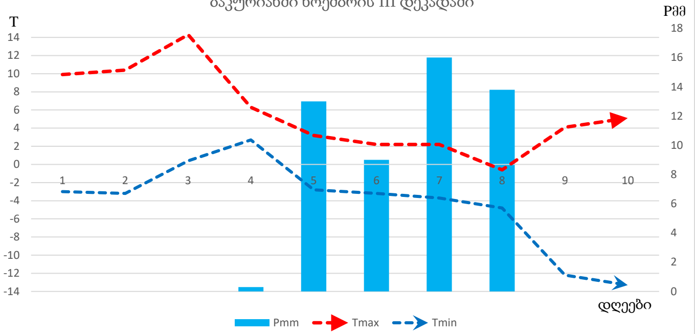
ჰაერის ტემპერატურის (T) და ნალექების (Pმმ) მსვლელობა ბაკურიანში ნოემბრის III დეკადაში
