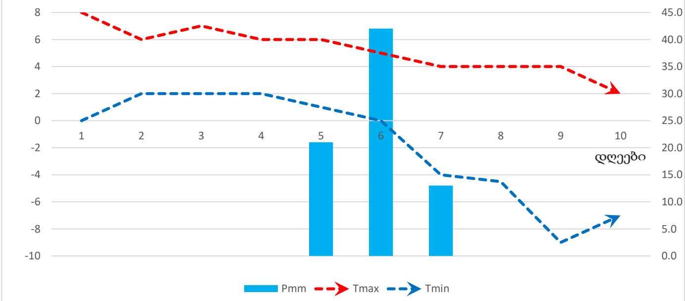
ჰაერის ტემპერატურის (T) და ნალექების (Pმმ) მსვლელობა გულდაურში ნოემბრის III დეკადაში
